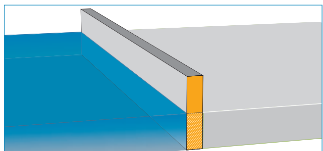
17 Unterirdische Abdichtung einer Schutzschwelle
