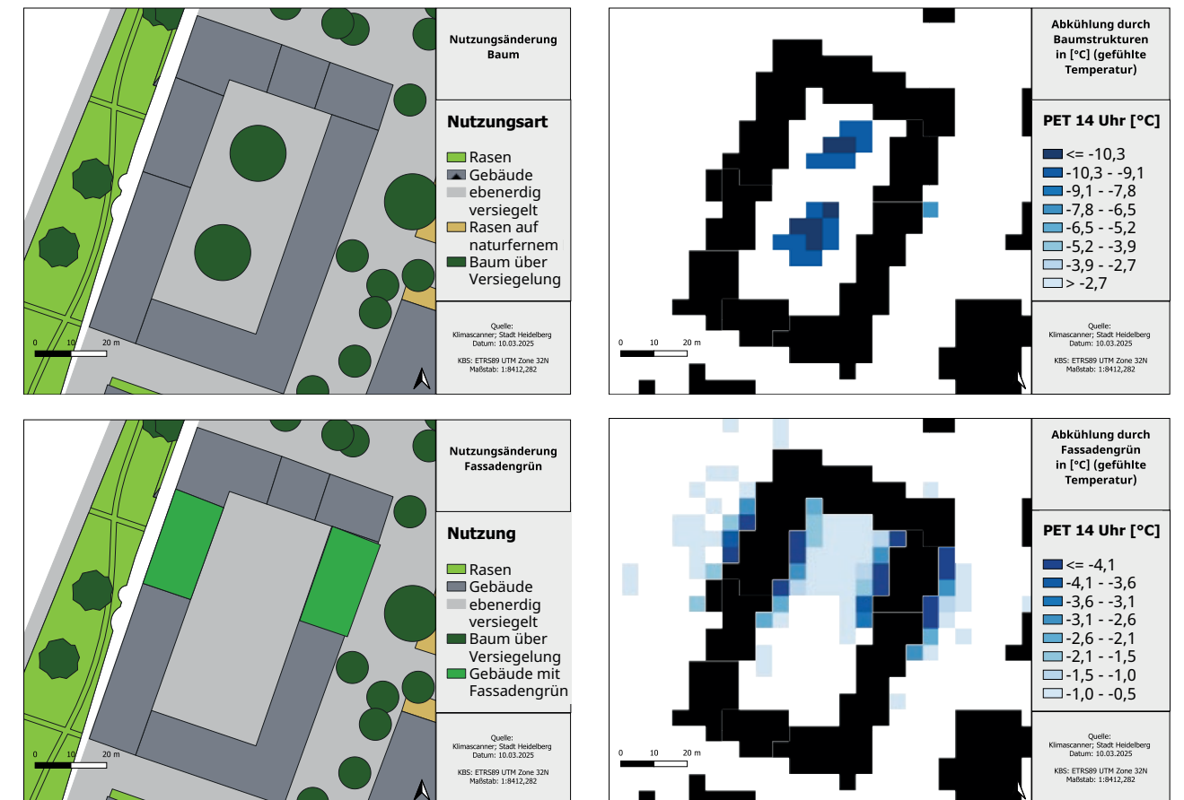
Abb. 2: Wirkung von Baumpflanzung (oben) und Fassadenbegrünung (unten) in einem idealisierten Baublock
