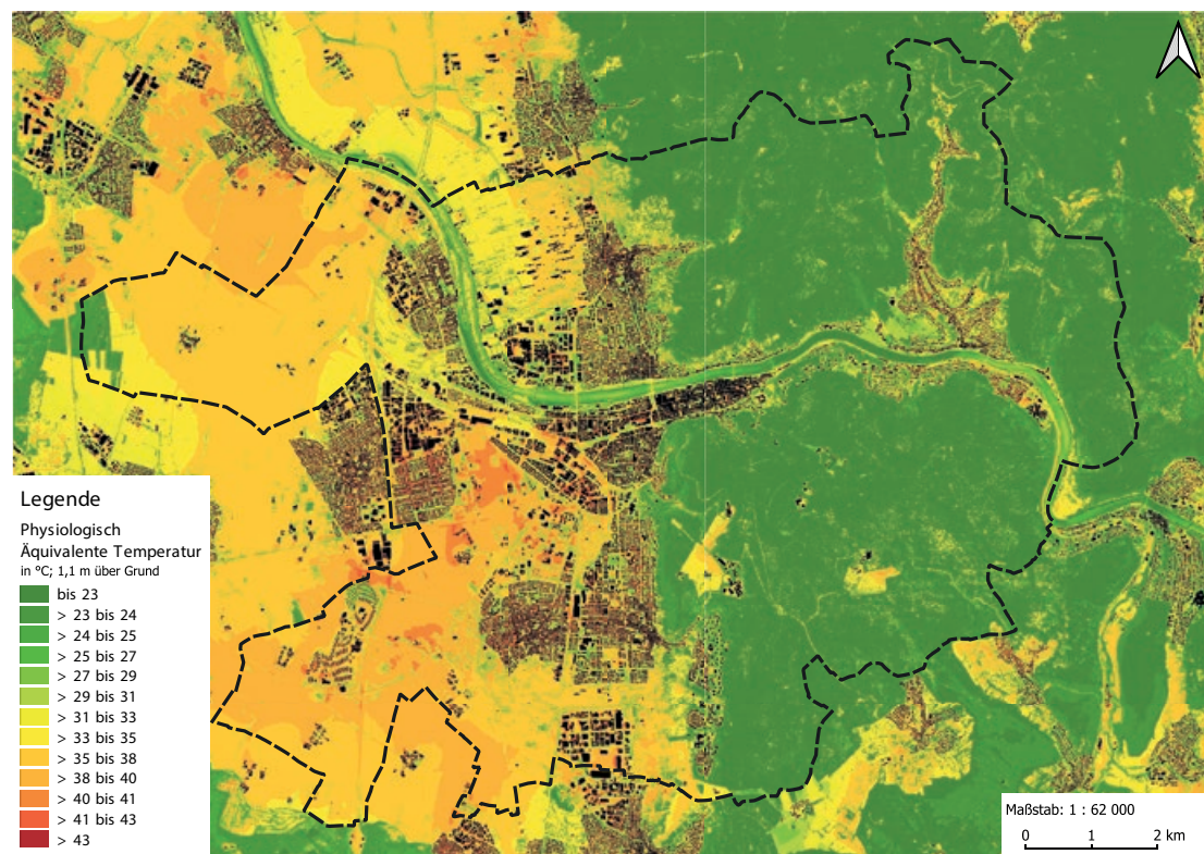
Abb. 1. Die Karte zeigt die berechnete physiologische Äquivalenztemperatur [°C] 1,1 m über Grund für einen heißen Sommertag um 14:00 UTC. Die physiologisch äquivalente Temperatur (PET) ist ein Maß für die gefühlte Temperatur beziehungsweise die Wärmebelastung. Orange bis rote Flächen in der Abbildung zeigen Teilbereiche mit hoher Wärmebelastung. Hier wird vor allem auch deutlich, dass freiliegende trockene Ackerflächen bei starker Hitze und Trockenheit nahezu keine Kühlfunktion aufweisen. Grüne Bereiche zeigen kühlere Standorte
